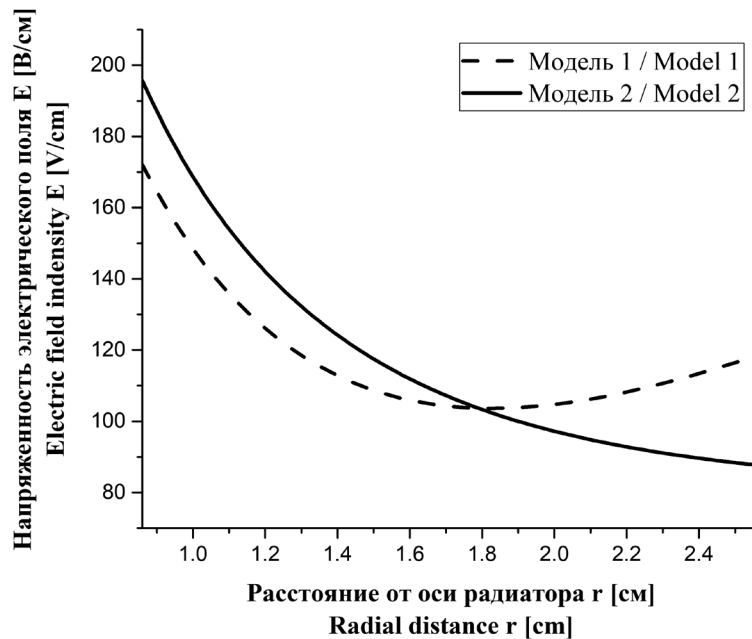
Рис. 4. Радиальная зависимость электрического поля
