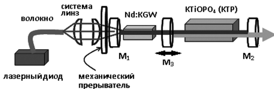
Рис. 1. Схема Nd:KGdW/КТП-лазера с внутрирезонаторным удвоением частоты
